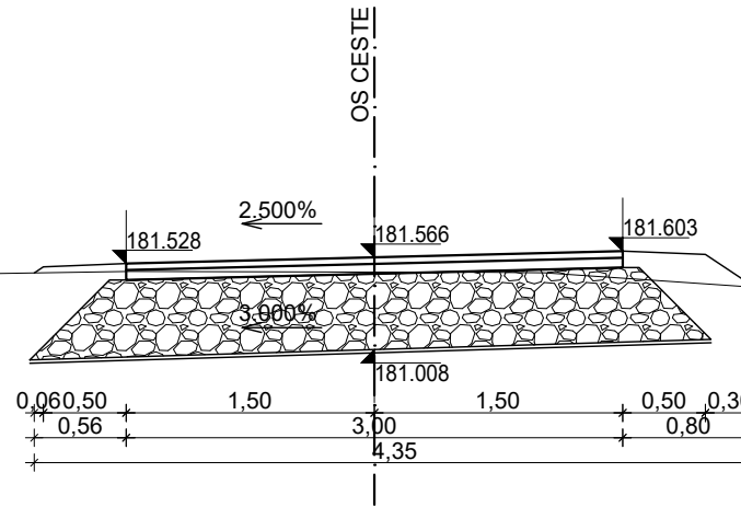
KARAKTERISTIČNI POPREČNI PRESJEK 3 stac. 0+060.00 km
