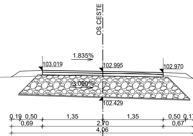
KARAKTERISTIČNI POPREČNI PRESJEK 2 stac. 0+040.00 km
