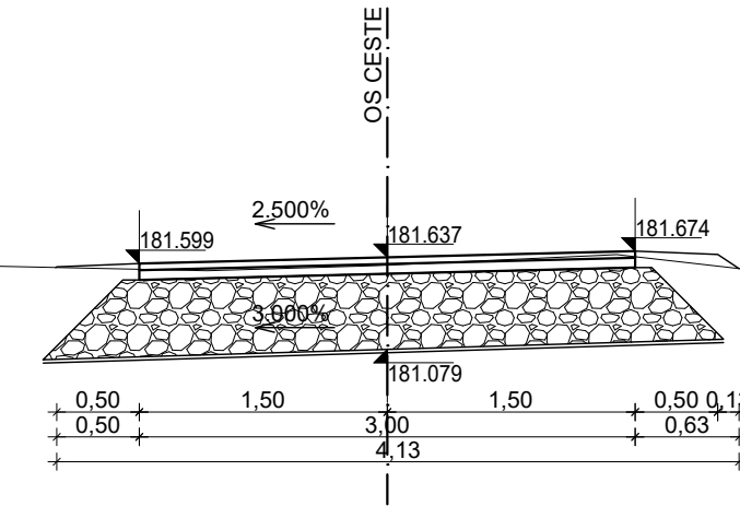
KARAKTERISTIČNI POPREČNI PRESJEK 1 stac. 0+020.00 km
