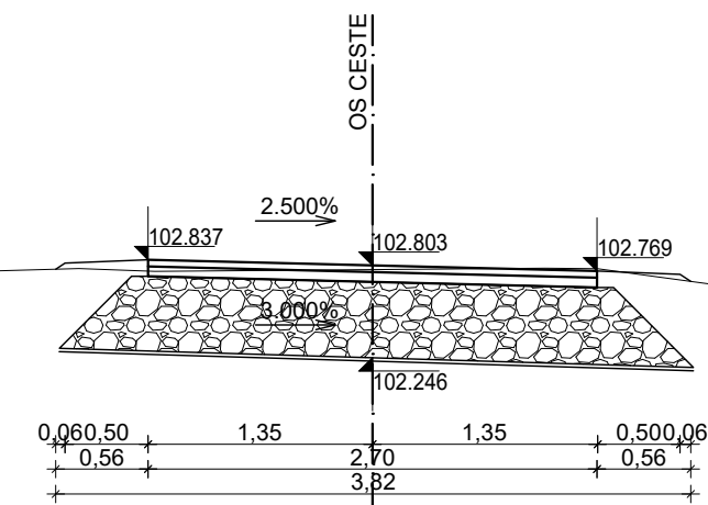
KARAKTERISTIČNI POPREČNI PRESJEK 1 stac. 0+020.00 km
