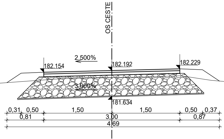
KARAKTERISTIČNI POPREČNI PRESJEK 5 stac. 0+100.00 km
