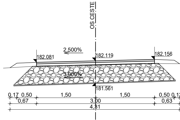
KARAKTERISTIČNI POPREČNI PRESJEK 6 stac. 0+120.00 km
