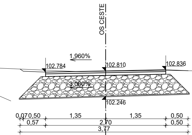
KARAKTERISTIČNI POPREČNI PRESJEK 6 stac. 0+120.00 km
