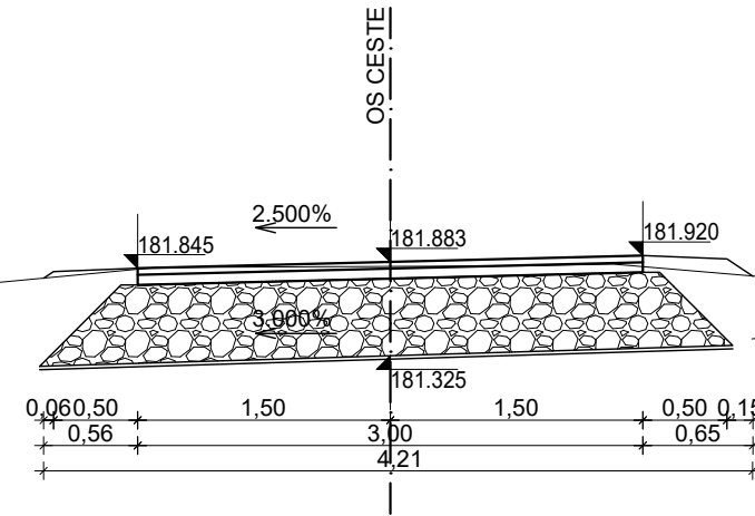
KARAKTERISTIČNI POPREČNI PRESJEK 4 stac. 0+080.00 km
