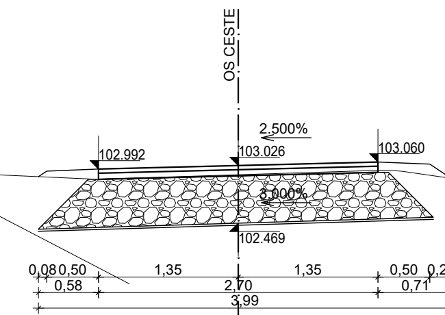
KARAKTERISTIČNI POPREČNI PRESJEK 4 stac. 0+080.00 km
