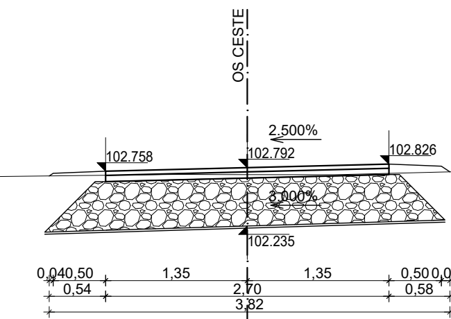
KARAKTERISTIČNI POPREČNI PRESJEK 5 stac. 0+100.00 km
