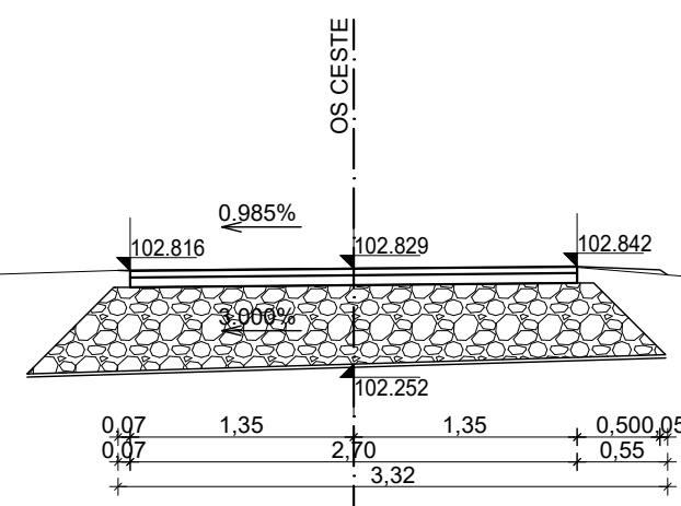
KARAKTERISTIČNI POPREČNI PRESJEK 7 stac. 0+140.00 km
