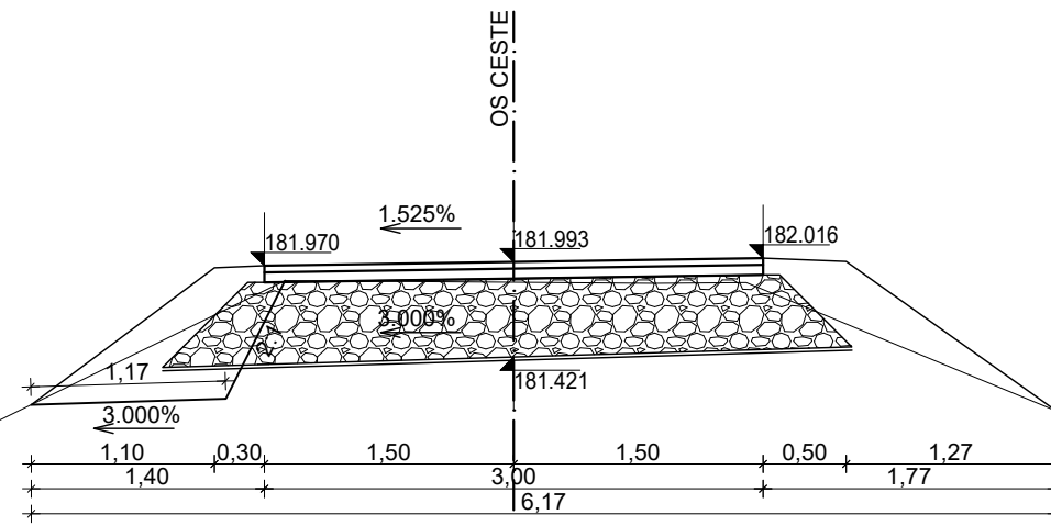
KARAKTERISTIČNI POPREČNI PRESJEK 7 stac. 0+140.00 km
